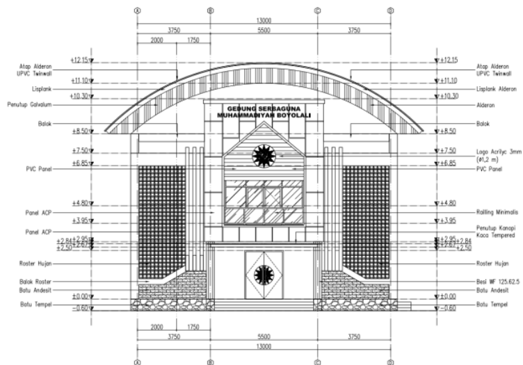
Gambar 4. Detail Arsitektur Tampak Depan.
