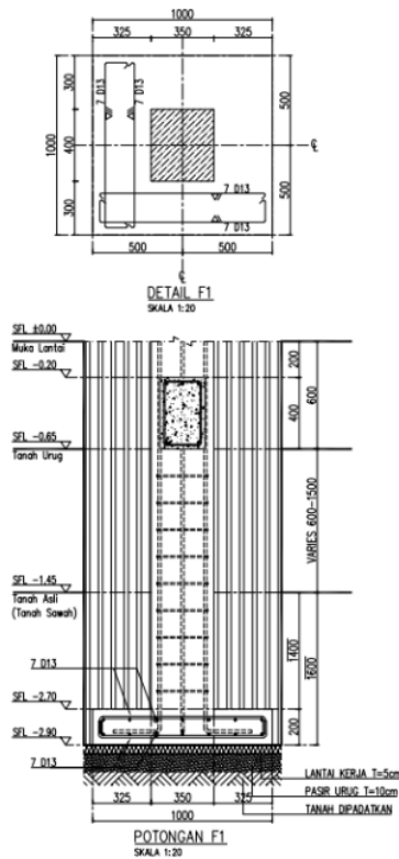
Gambar 6. Detail Penulangan Pondasi.
