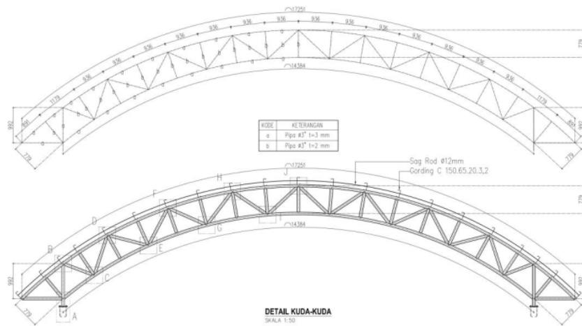
Gambar 5. Detail Struktur kuda-kuda.
