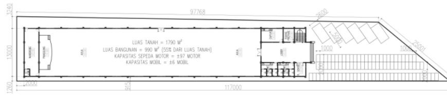
Gambar 2. Denah Gedung Serbaguna.
